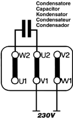
Motore 4 poli • Motor 4 poles • Motor 4 polig • Moteur 4 pôles • Motores 4 polos
