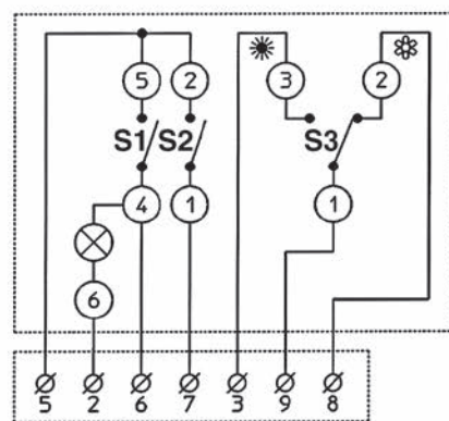
Comando a distanza Cod. 9015025
