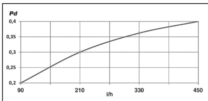
Modèle DN 20
