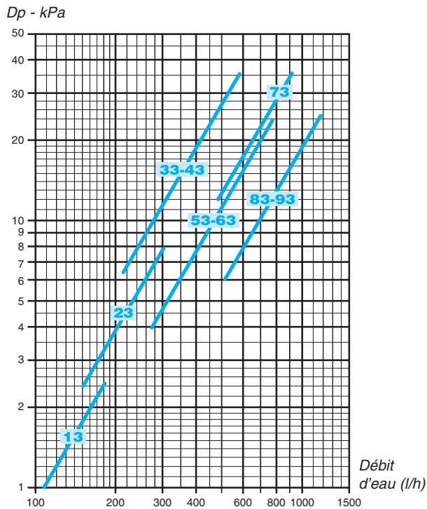
Batterie 3 rangs
