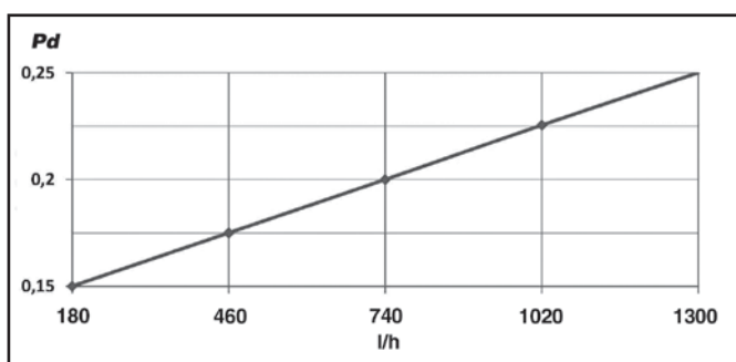
Modèle DN 20
