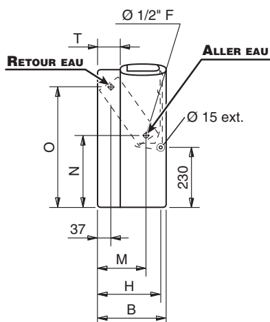
Batterie à 3 ou 4 rangs
