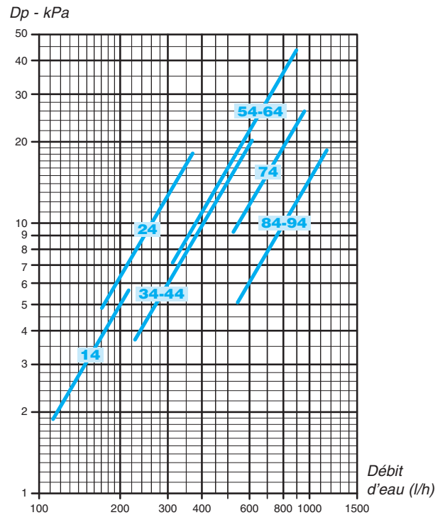
Batterie 4 rangs
