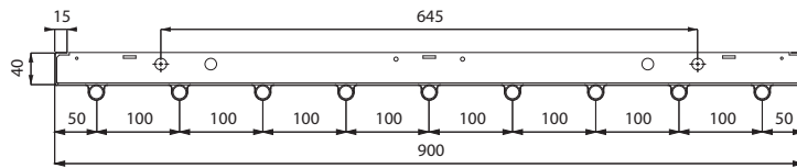
DS-ST18-3-120; 12 PIPES
