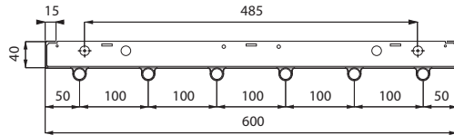
DS-ST18-3-090; 9 PIPES
