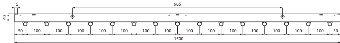
DS-ST18-3-150; 15 PIPES
