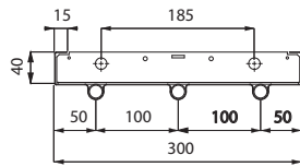
DS-ST18-3-060; 6 PIPES
