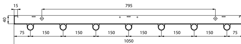
DS-ST28-2-120; 8 TUBI
