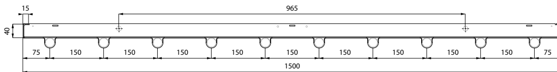
DS-ST28-2-150; 10 TUBI
