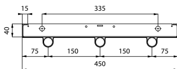
DS-ST28-2-060; 4 TUBI
