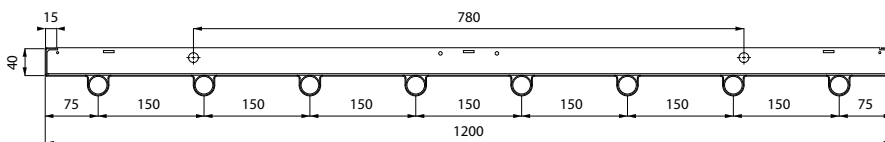
DS-ST28-2-135; 9 TUBI
