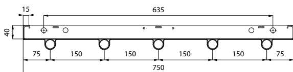
DS-ST28-2-090; 6 TUBI
