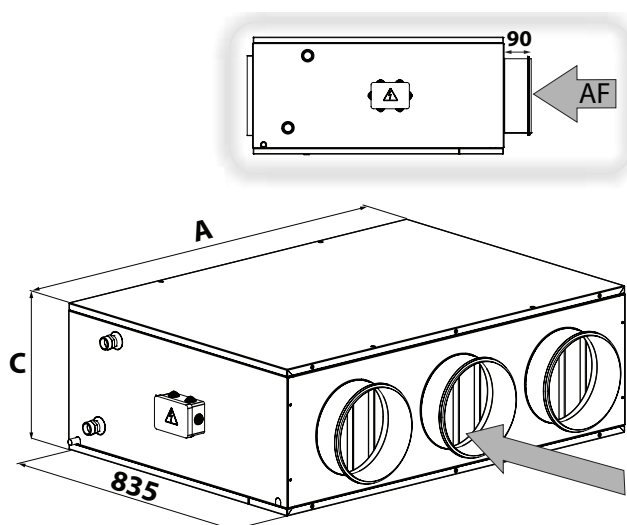
Vue débit d'air
