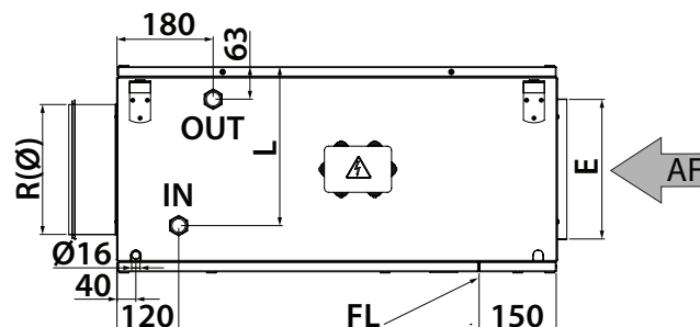
Version gauche (standard)
