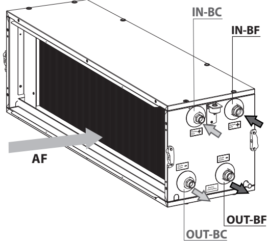
Raccords à droite (sur demande)
