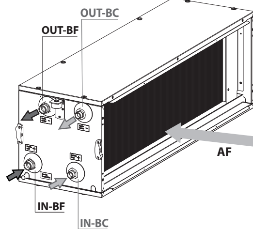
Raccords à gauche (standard)
