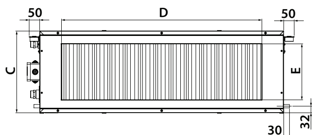
Vue côté filtre
