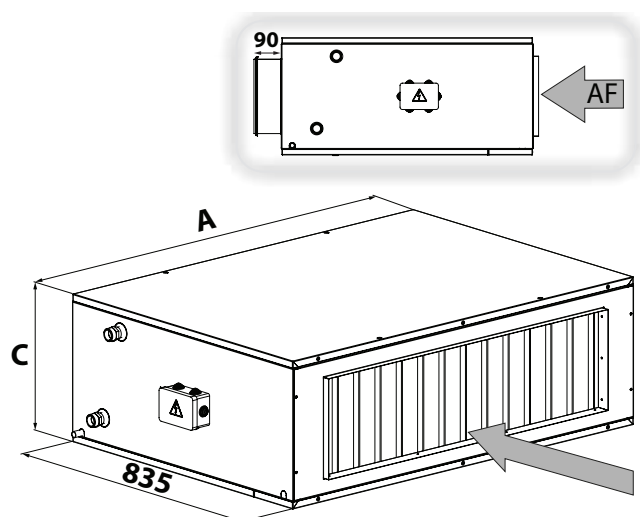
Vue débit d'air
