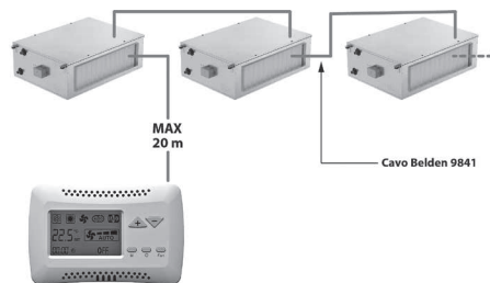
Une commande pour plusieurs unités (20 unités au maximum) (Longeur totale maxi du câble de raccordement = 800 m)
