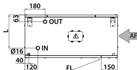
Version gauche (standard)
