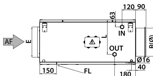
Version droite (sur demande)
