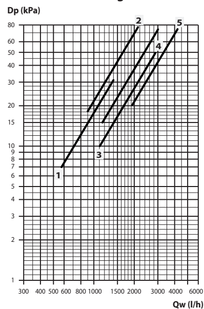
Batterie additionnelle à 2 rangs
