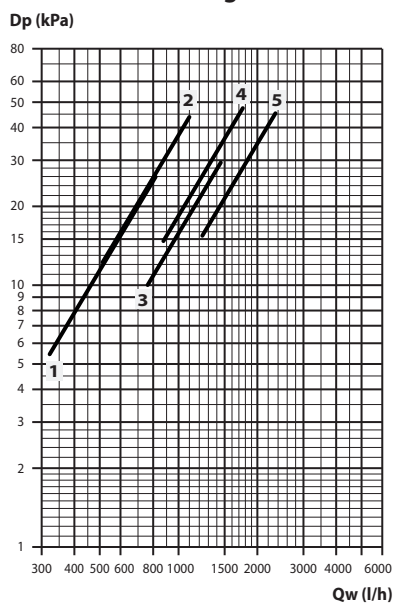
Batterie additionnelle à 1 rang
