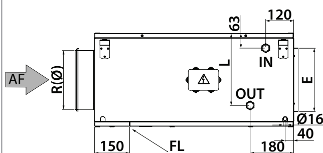
Version droite (sur demande)
