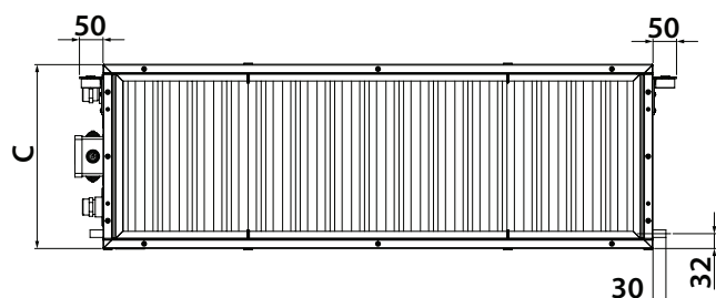
Vue côté filtre
