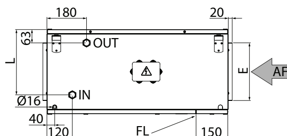
Version gauche (standard)
