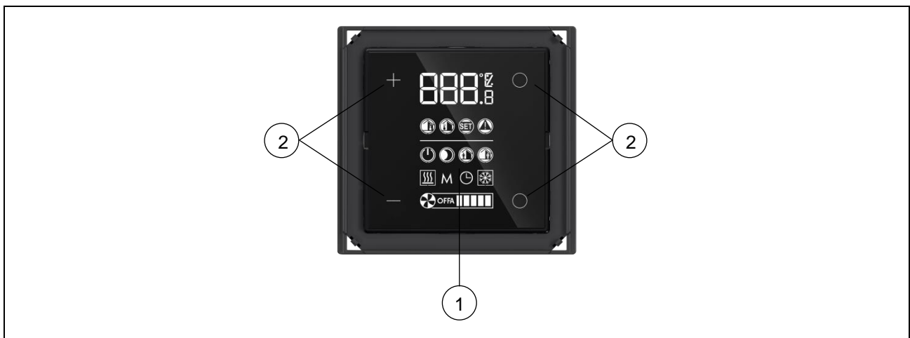
Interfaccia utente: display LCD (1), pulsanti di tipo capacitivo (2)
