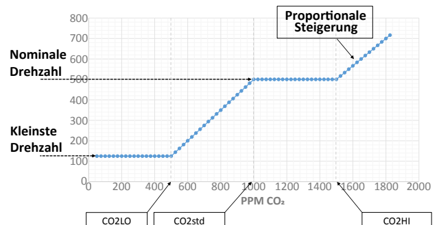
GRAFIK STEUERUNGSLOGIK DER LUFTMENGE IN ABHÄNGIGKEIT VON PPM CO 2
