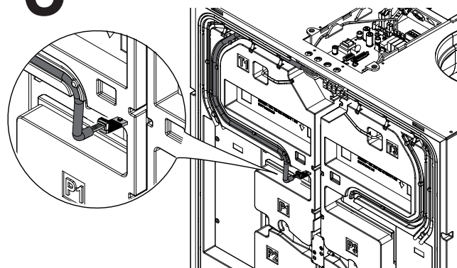
Posizione del sensore versione DESTRA (supplementare)
