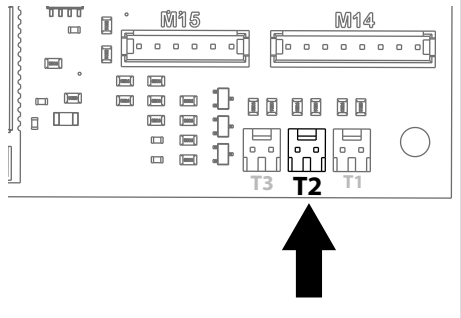
6.17 Collegamento sonda
