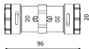
Articolo: SHRD01200120 x-light Raccordo diretto IR 20-20 mm
