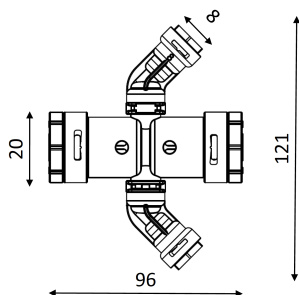
Articolo: SHTC02200208 x-light croce IR 2 ingressi 20x2 / 2 uscite 8x1 mm
