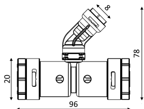
Articolo: SHTE02200108 x-light TEE IR 2 ingressi 20x2 / 1 uscita 8x1 mm
