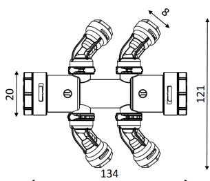
Articolo: SHTC02200408 x-light croce IR 2 ingressi 20x2 / 4 uscite 8x1 mm
