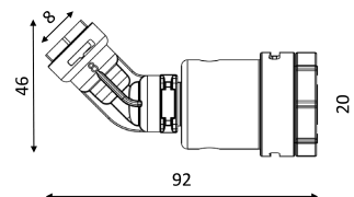
Articolo: SHRA01200108 x-light riduzione Angolare IR 20x2 mm & 8x1 mm
