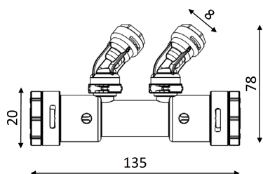
Articolo: SHTE02200208 x-light TEE IR 2 ingressi 20x2 / 2 uscite 8x1 mm
