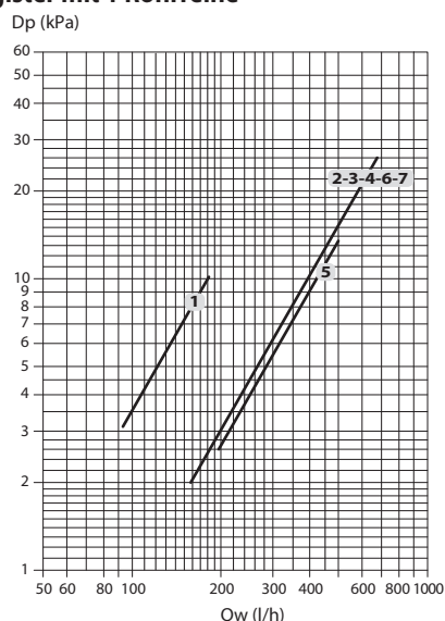
Zusatzregister mit 1 Rohrreihe
