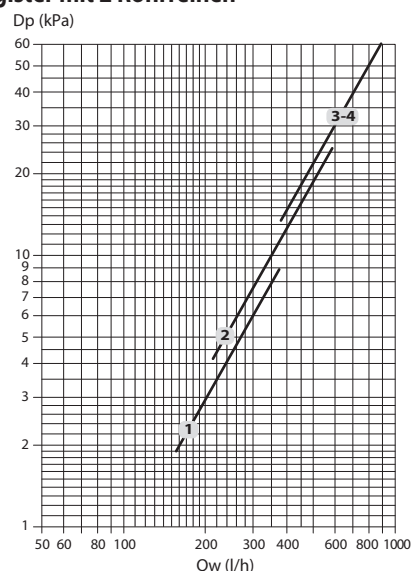
Zusatzregister mit 2 Rohrreihen
