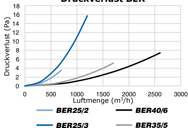
Druckverlust BER
