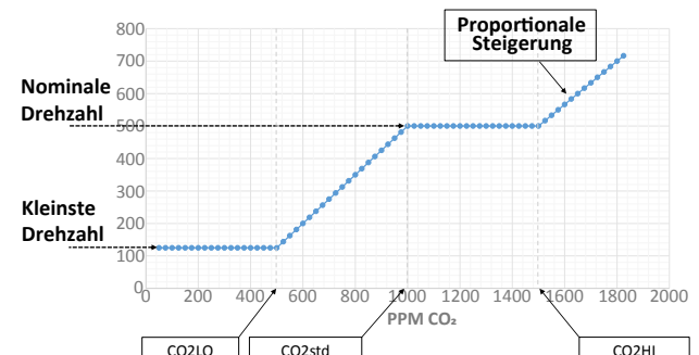
GRAFIK STEUERUNGSLOGIK DER LUFTMENGE IN ABHÄNGIGKEIT VON PPM CO 2
