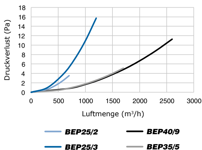
Druckverlust BEP
